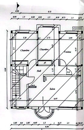
1er Etage A Construire
