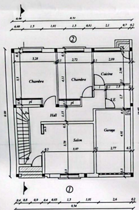
RDC Existant A Modifier
