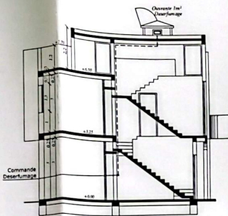
COUPE
